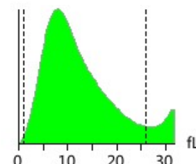
PLT Histogram
